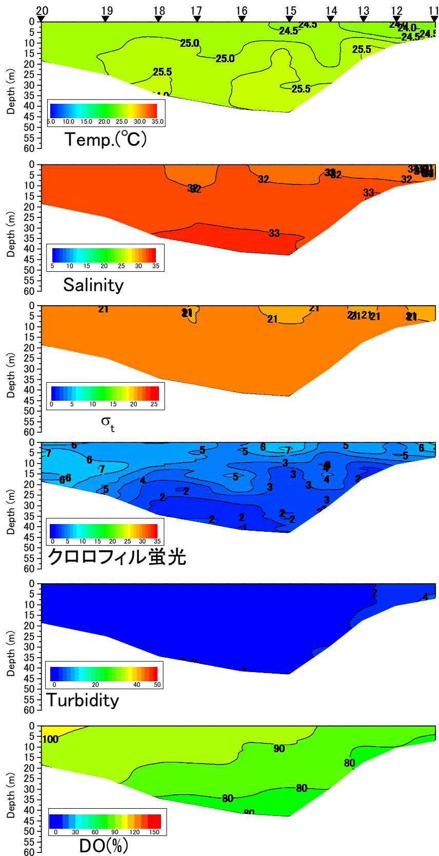
八代海中央ラインの水温(°C)、塩分、密度( \sigma_t )、クロロフィル蛍光強度、濁度、溶存酸素飽和度(DO%)の鉛直面図(国土交通省の調査による) (2016年10月13日)
